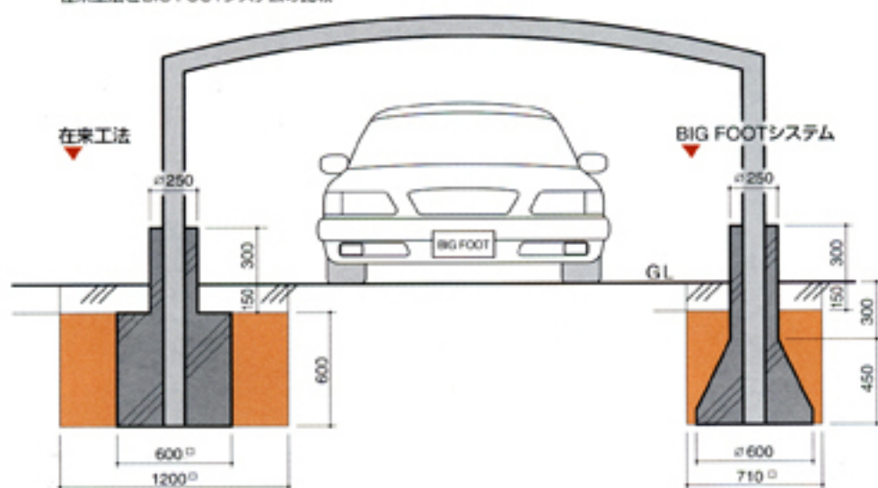
カーポートの基礎工事 施工図 在来工法とBIG FOOTシステムの比較
